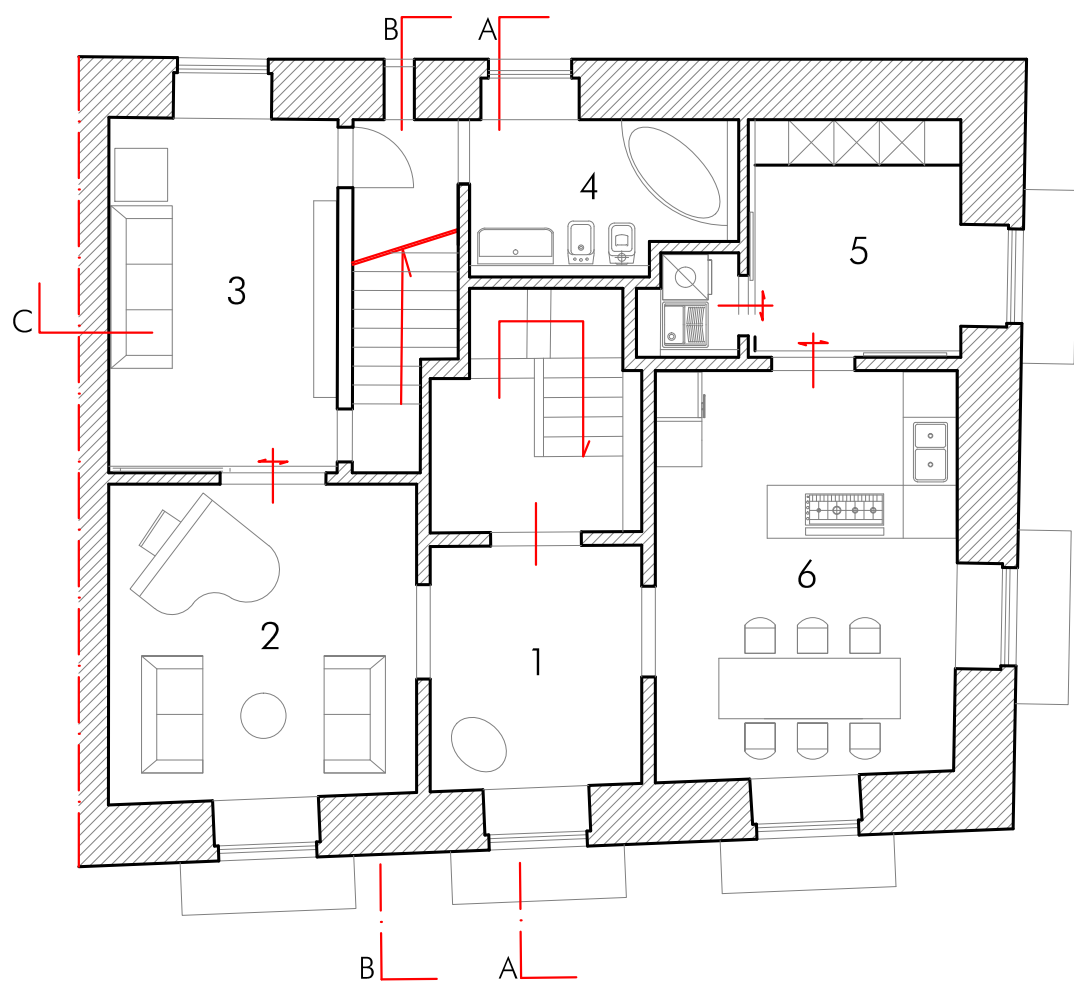
Planimetria Piano Primo
