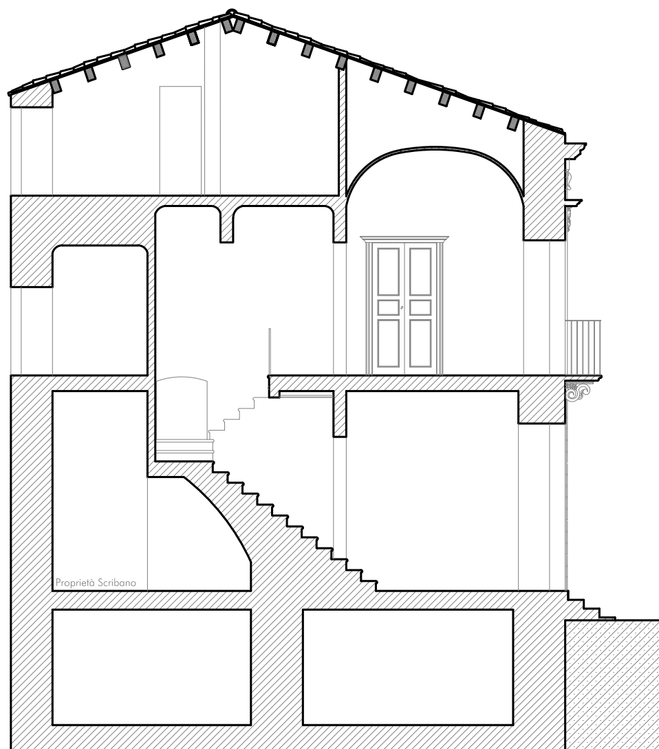
Sezione - Prospetto A - A
