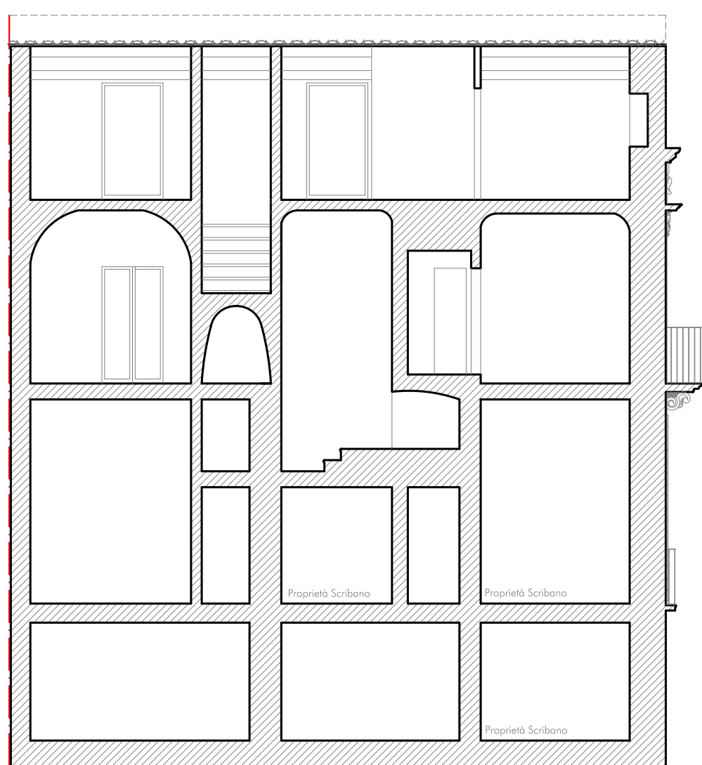
Sezione - Prospetto C - C
