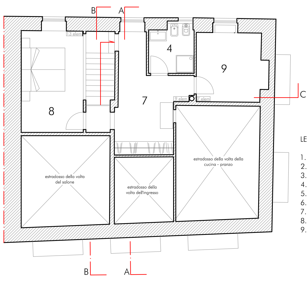
Planimetria Piano Sottotetto
