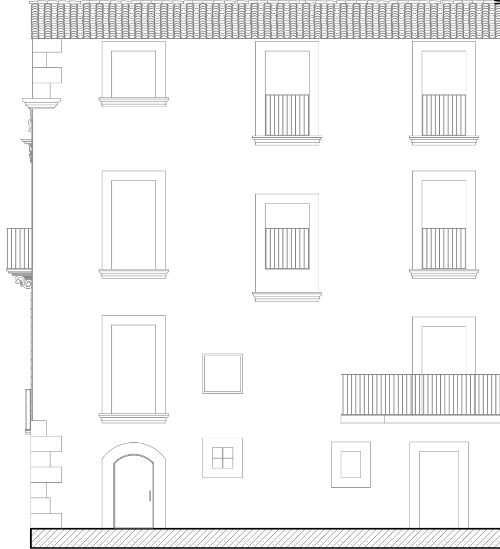
Prospetto Via Cardona
